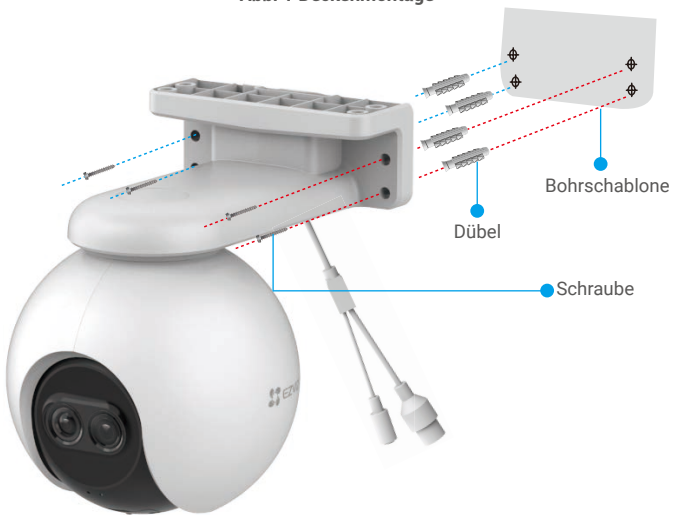
Abb. 2 Wandmontage
