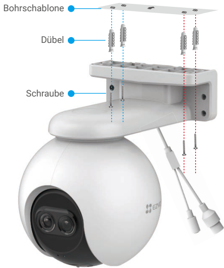
Abb. 1 Deckenmontage
